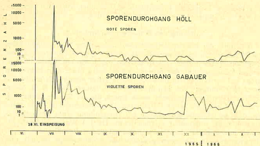
Abb. 5: Sporenaustritte beim Triftversuch Schlagerboden (Frankenfels, NÖ) 1965. Die in zwei Schwinden am 28. Juni eingespeisten Sporen (je 6 kg) traten voneinander getrennt in zwei verschiedenen Quellen aus. Der stärkste Austritt erfolgte nach wolkenbruchartigen Regenfällen erst am 19. Juli (Höllquelle: 16.400 rote Sporen) und am 20. Juli (Gabauerquelle: 17.900 violette Sporen). Die Sporenaustritte klangen langsam ab. Im Dezember wurde nach starken Niederschlägen in der Gabauerquelle neuerlich ein starker Sporenaustritt (1670 Sporen) festgestellt. Im Februar 1966 lieferten beide Quellen noch bedeutende Sporenmengen (Höllquelle: 5—20 Sporen pro Probe; Gabauerquelle: 10—400 Sporen pro Probe). Die Horizontalentfernung und der Höhenunterschied zwischen Schwinde und Quelle betragen beim Triftweg zur Höllquelle 1 km bzw. 40 m und beim Triftweg zur Gabauerquelle 1,3 km bzw. 110 m. Über die Detailergebnisse dieses Versuches wird an anderer Stelle berichtet werden.
