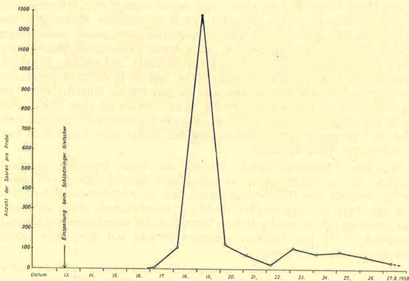
Abb. 4: Der Sporendurchgang im Waldbachursprung beim Triftversuch Dachstein 1958 als Beispiel für eine geschlossene Triftung der Hauptsporenmenge von einer starken Schwinde (Gletscherschwinde > 5 l/s) zu einer Riesenquelle ( > 1 m 3 /s). Die Horizontalentfernung zwischen Schwinde und Quelle beträgt 8,4 km, der Höhenunterschied 1480 m. (Aus J. ZÖTL 1960/61). Der Durchgang konnte durch 24stündige Probenentnahme noch sehr gut erfaßt werden.
