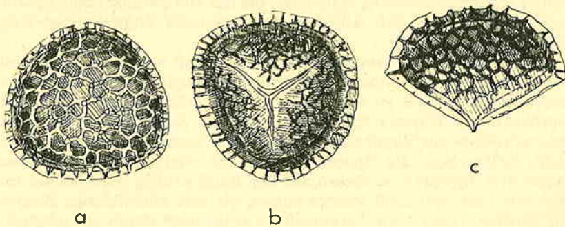
Abb. 1: Sporen von Lycopodium clavatum nach G. ERDTMAN (1954). Erläuterungen siehe im Text.
